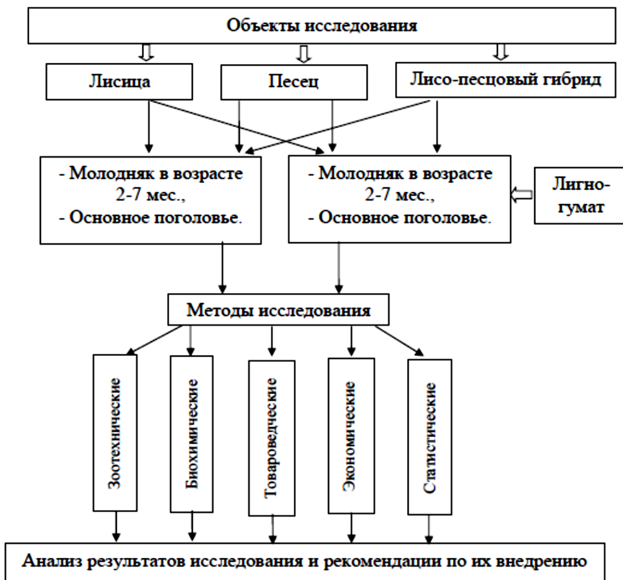
Рис. 1. Схема исследования
